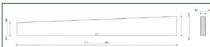
Viga cónica
