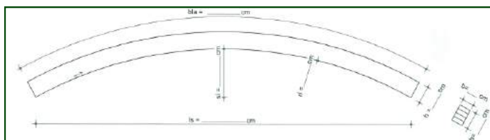
Viga curva
