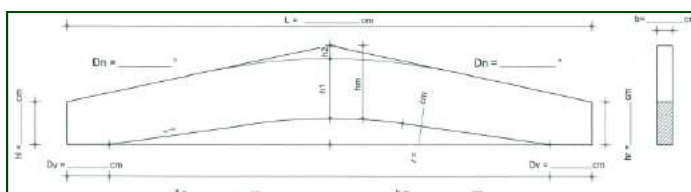
Viga peraltada con cordón inferior doblado
